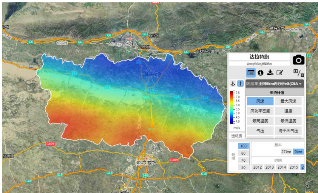
图 2 达拉特旗风资源分布图
